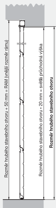
Montáž za ostění
