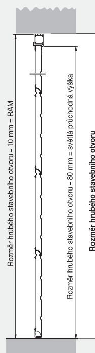
Montáž do ostění
